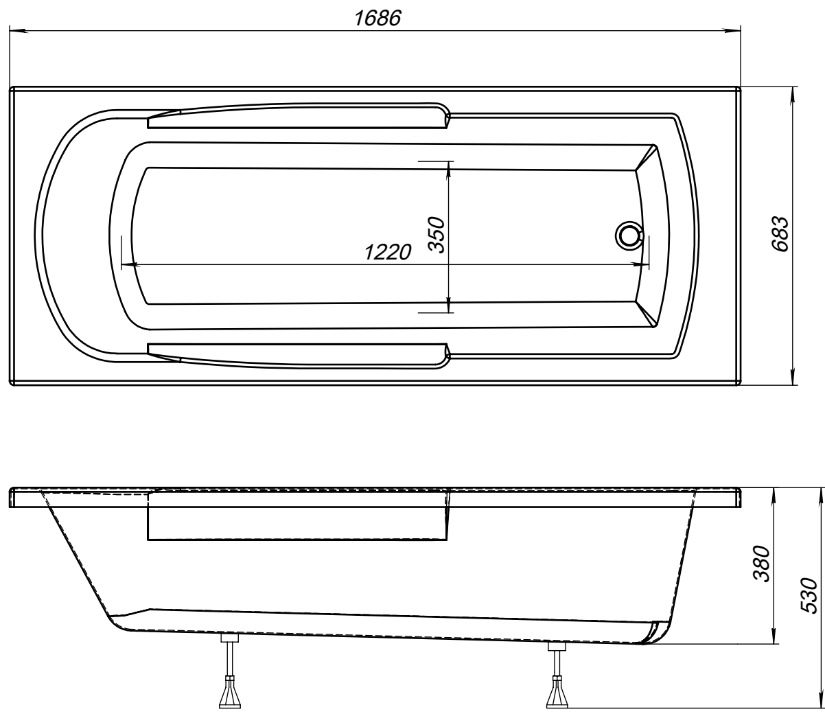
Ванна 170x70 - Extra - Схема с габаритными размерами Объем 190 лит. (уровень воды 75 мм от верхнего борта)
