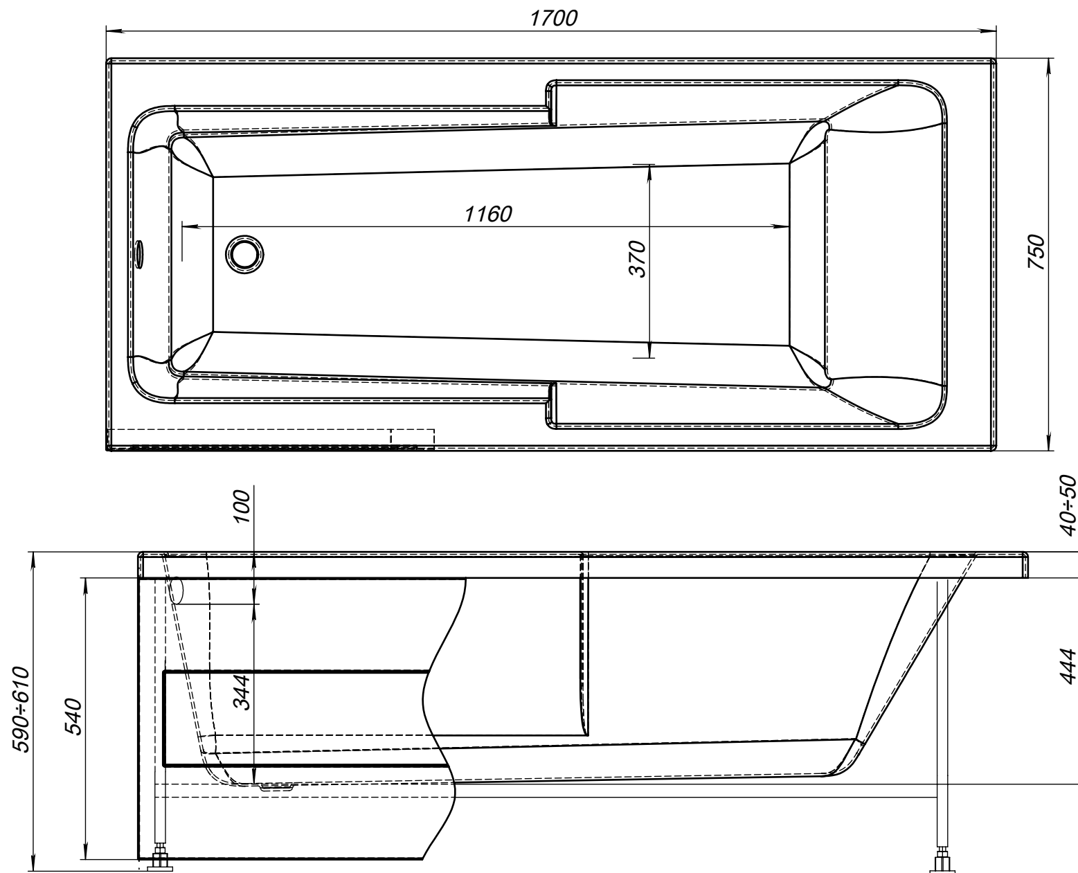
Ванна 170x75 - Taurus - Схема с габаритными размерами Объем 200 лит. (уровень воды 100мм от верхнего борта)
